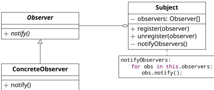
UML-диаграмма классов для шаблона Observer
